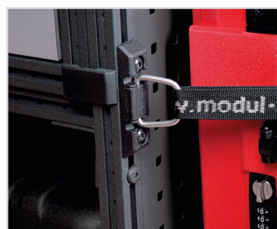
Kiinnityssilmukka T-uraan
